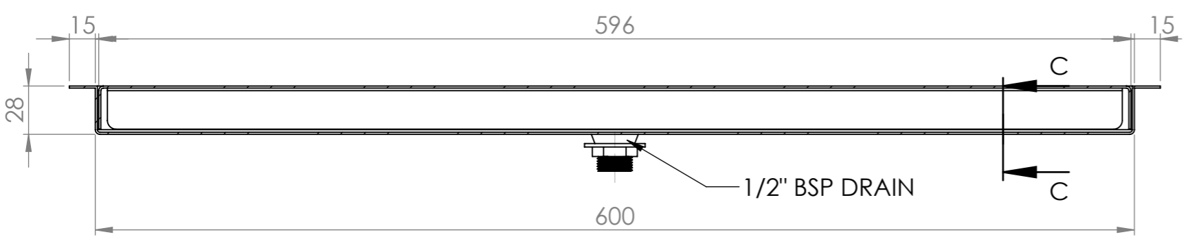
SECTION A-A
